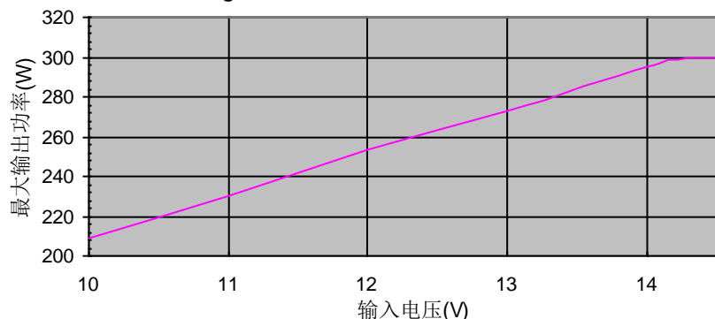
iCharger1010B+: 最大输出功率 与 输入电压 关系图
