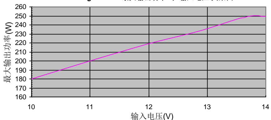
iCharger106B+：最大输出功率与输入电压关系图
